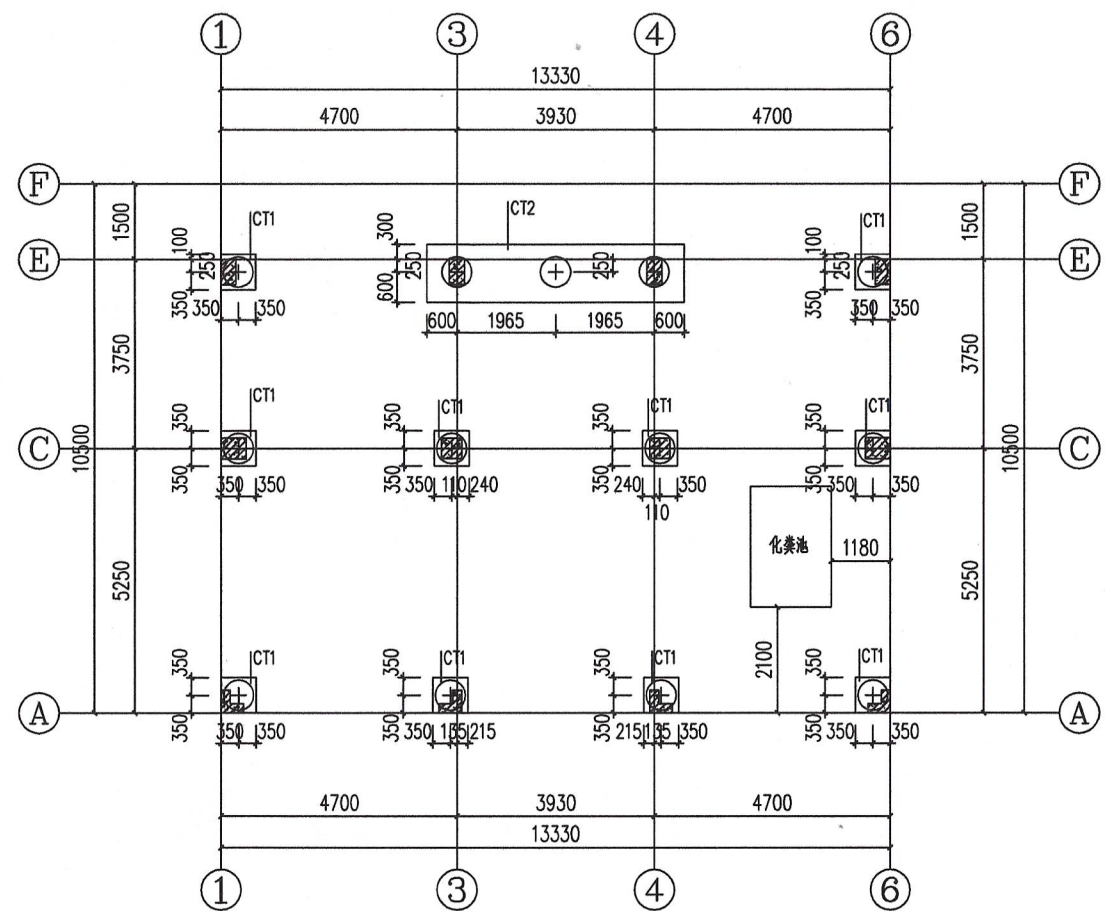
桩基承台平面布置图
